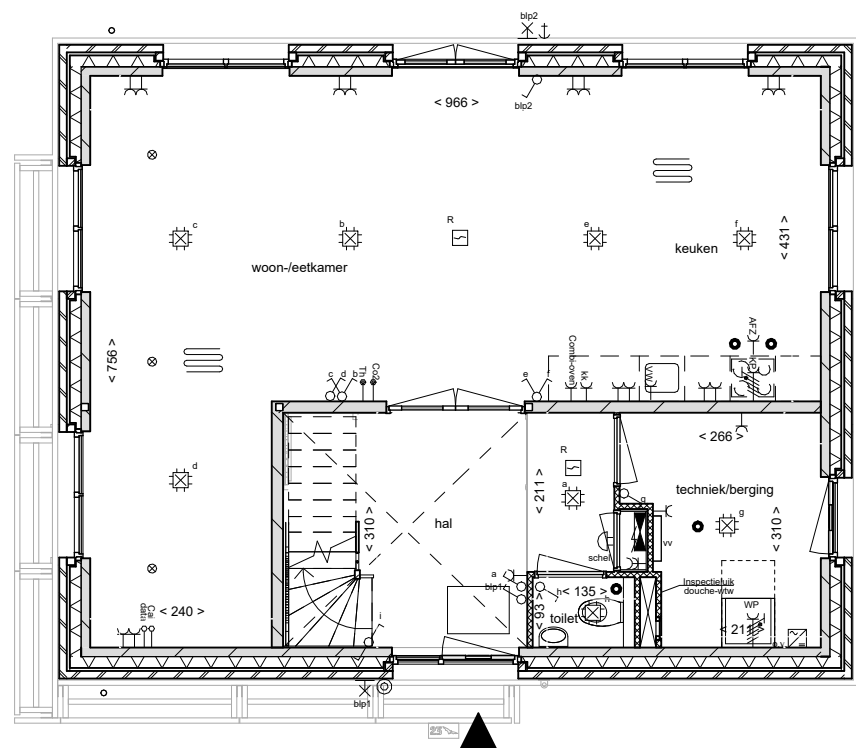
begane grond
