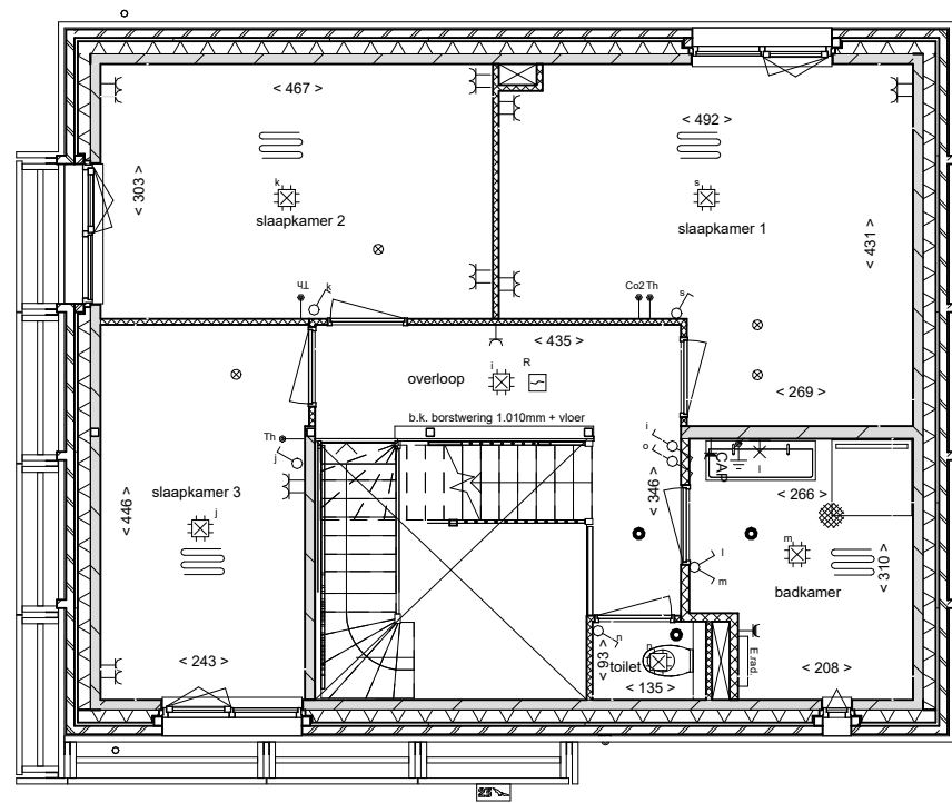
eerste verdieping
