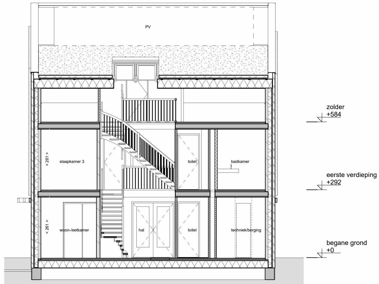
Doorsnede A
