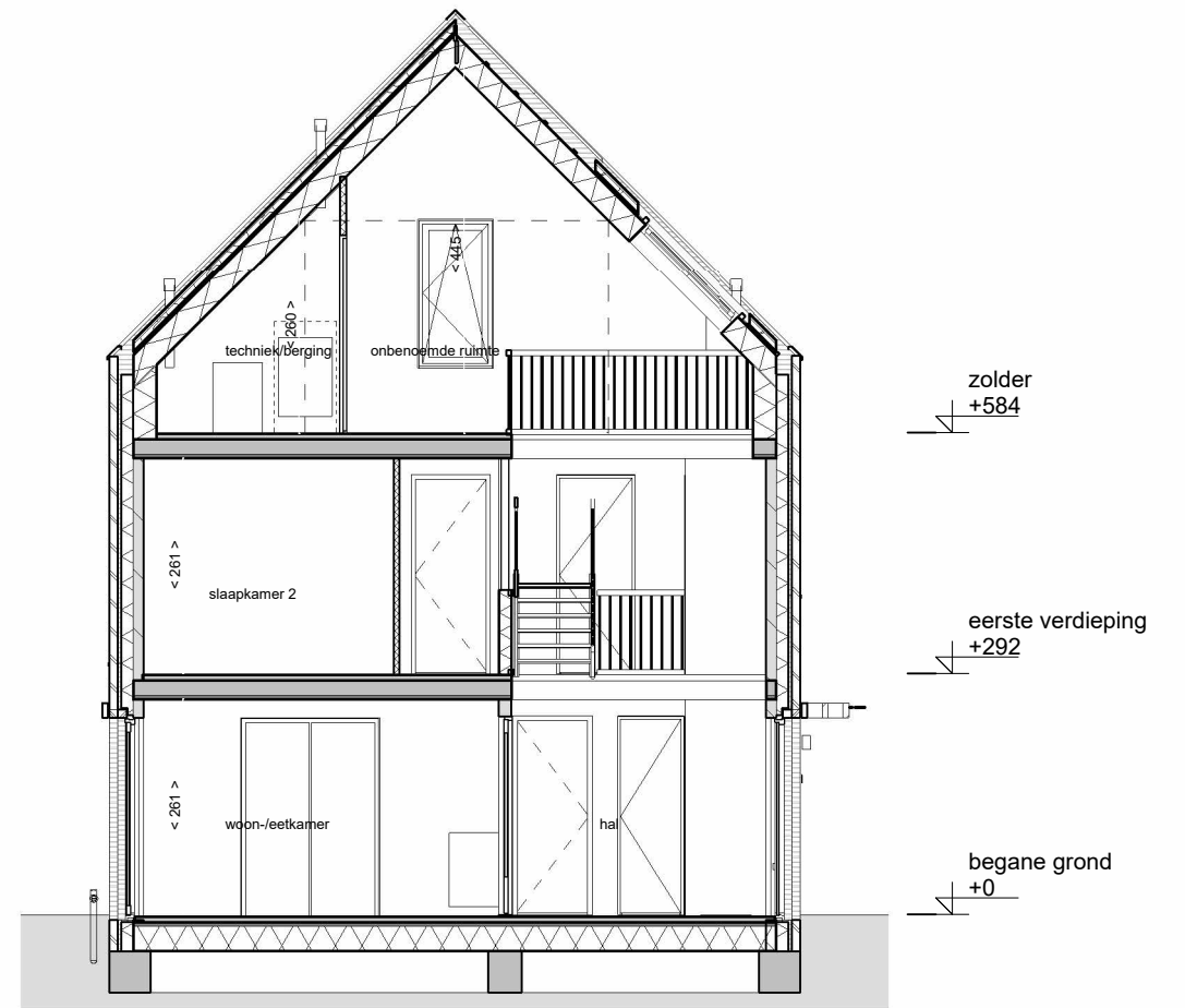
Doorsnede B
